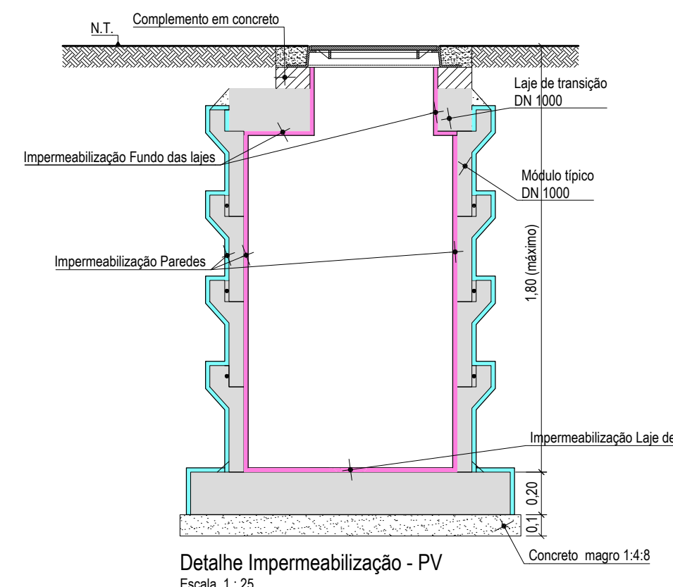
Detalhe Impermeabilização - PV Escala 1:25
