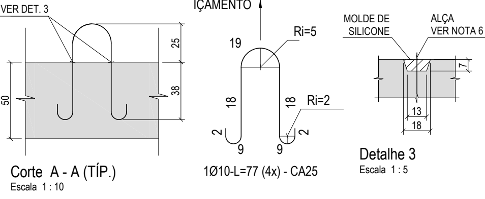
Corte A - A (TÍP.) Escala 1:10
