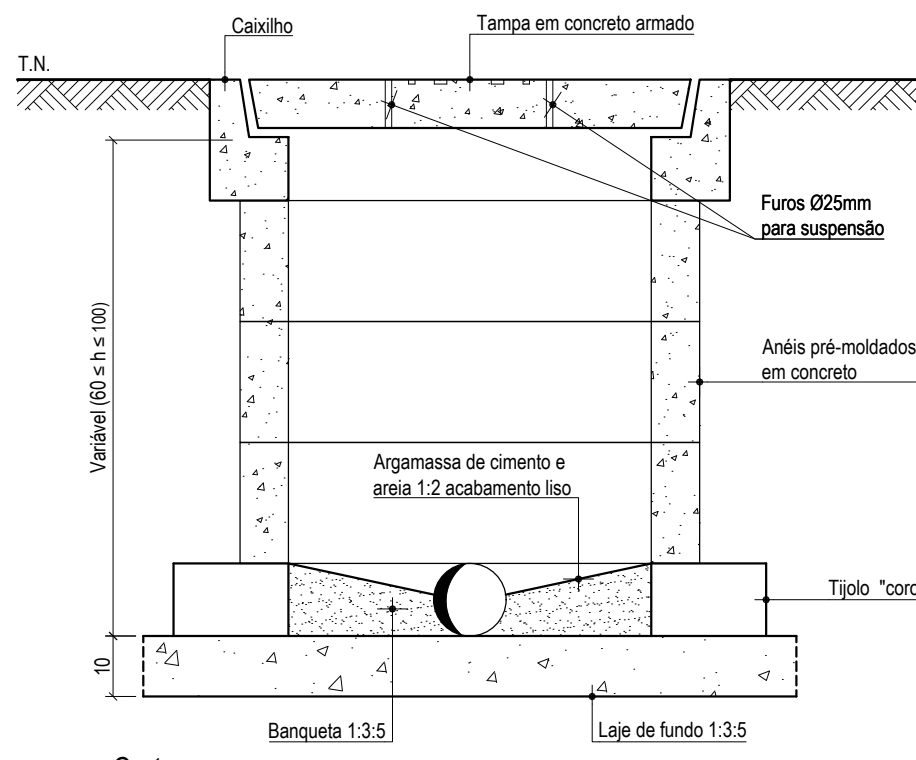
Corte Escala 1:12,5
