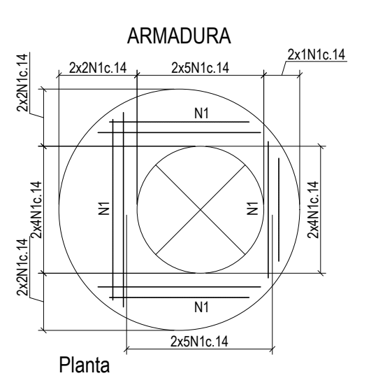
Planta Escala 1:25
