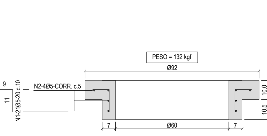
Anel de Ajuste - PV DN 600 (Ponta e Bolsa) Escala 1:10
