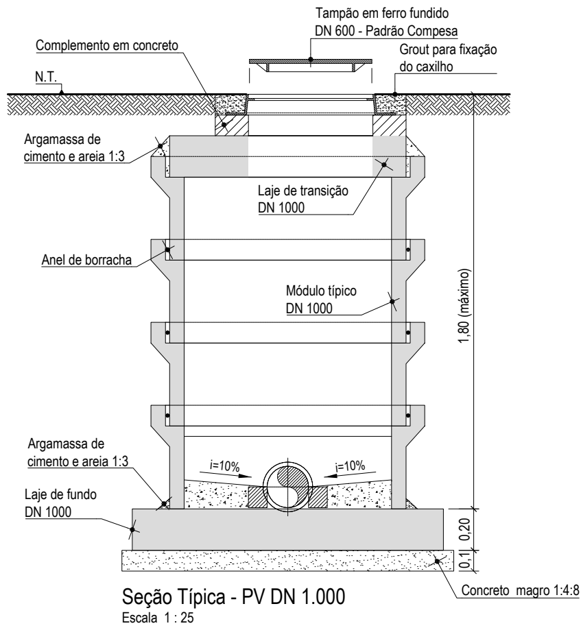
Seção Típica - PV DN 1.000 Escala 1:25
