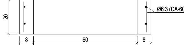
Detalhe do Anel - Corte Escala 1:12,5
