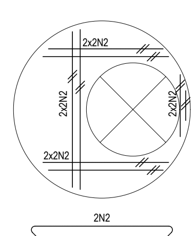
Planta Escala 1:25
