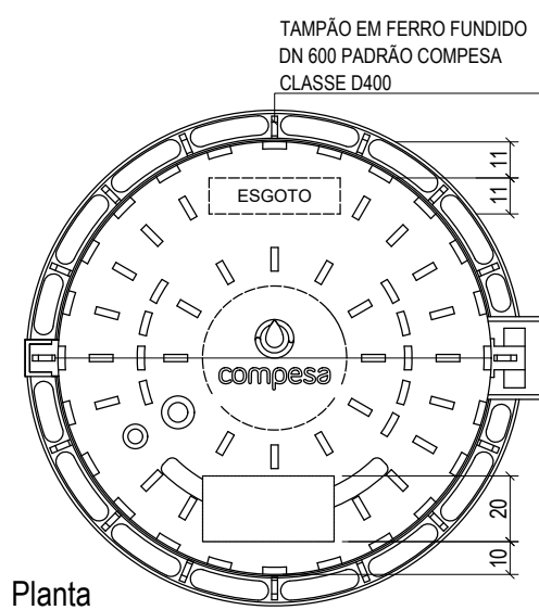
Planta Escala 1:12,5
