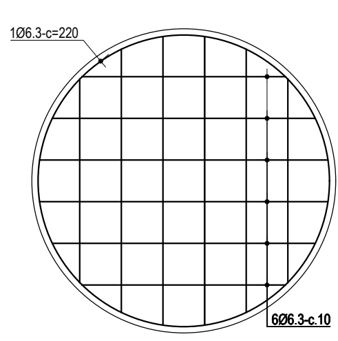
Detalhe da Tampa - Planta Escala 1:12,5
