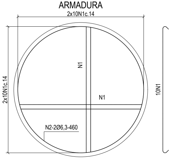
Planta Escala 1:25
