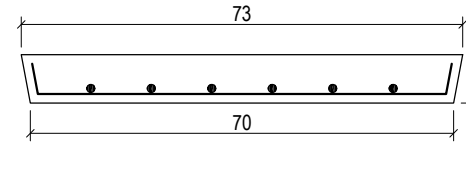
Detalhe da Tampa - Corte Escala 1:12,5
