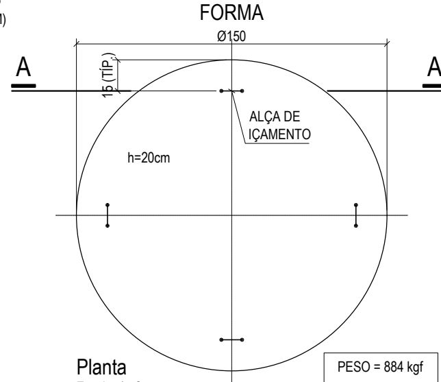
Planta Escala 1:25
