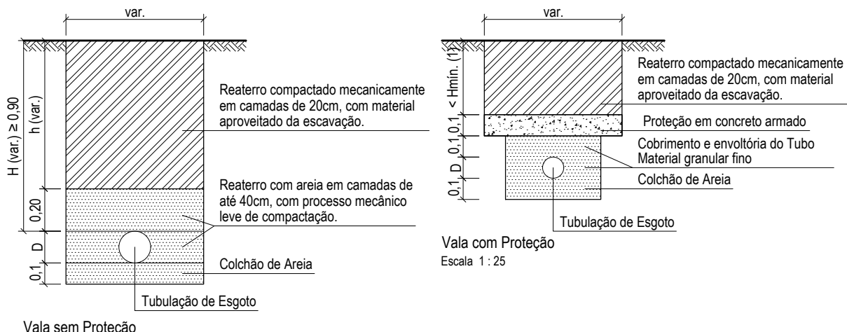
Vala sem Proteção Escala 1:25
