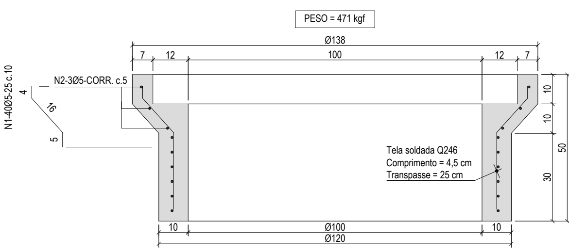
Módulo Típico - PV DN 1.000 (Ponta e Bolsa) Escala 1:12,5
