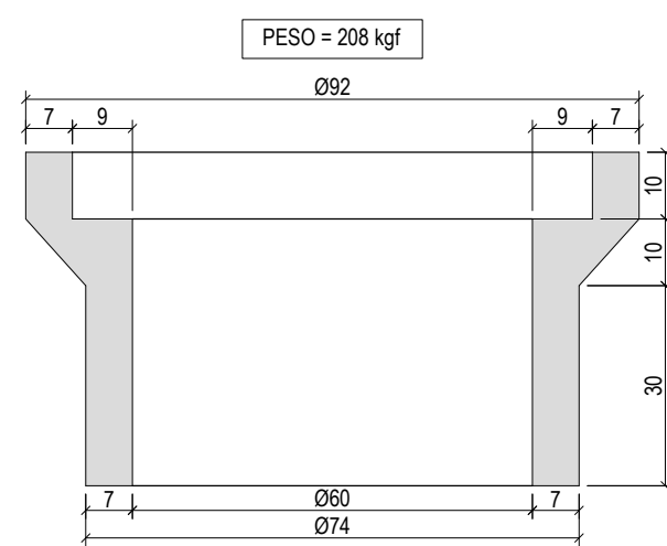
Módulo Típico - PV DN 600 (Ponta e Bolsa) Escala 1:10
